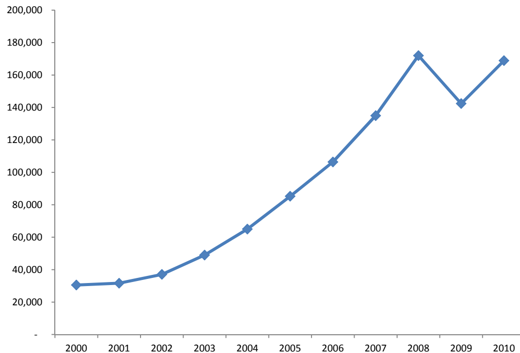
Graphique : évolution du PIB de la CEEAC entre 2000 et 2010 (en millions de USD)
